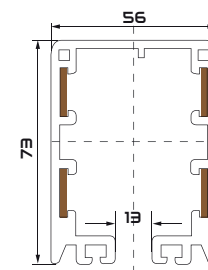
4P:35A-240A
