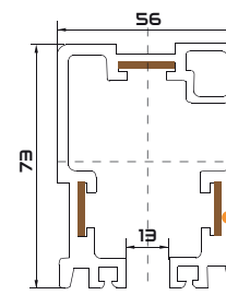
3P:35A-170A
